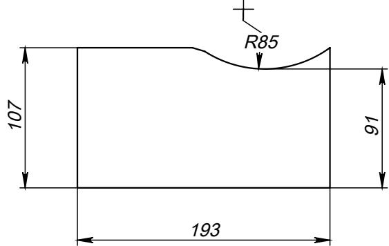
Поз.2 (Угольник) развертка
