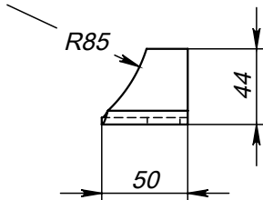
Поз.5 (Ушко)
