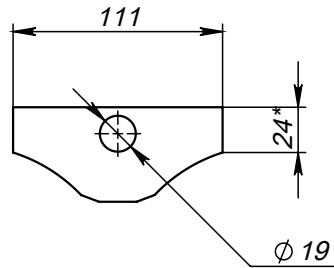
Поз.5 (Ушко) развертка
