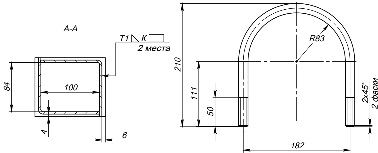
Поз.4 (Хомут)
